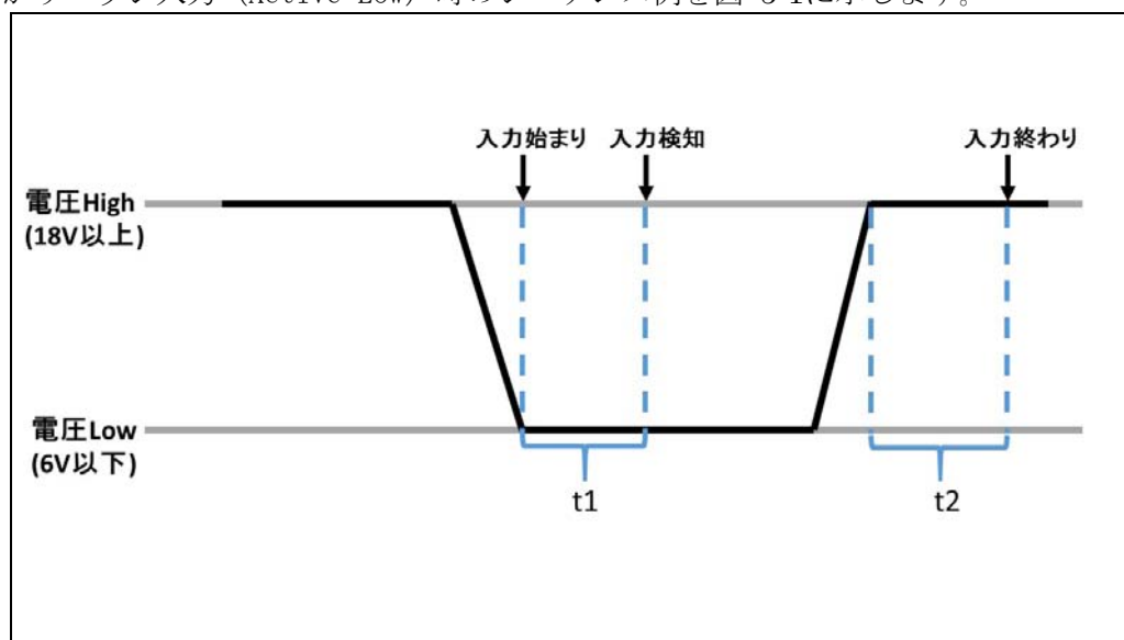
図 5-1 立ち下がりエッジ入力（Active Low）時のシーケンス図
