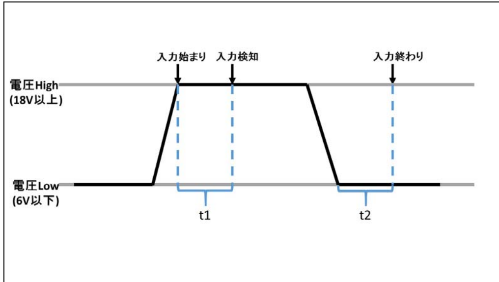
図 5-2 立ち上がりエッジ入力 (Active High) 時のシーケンス図
