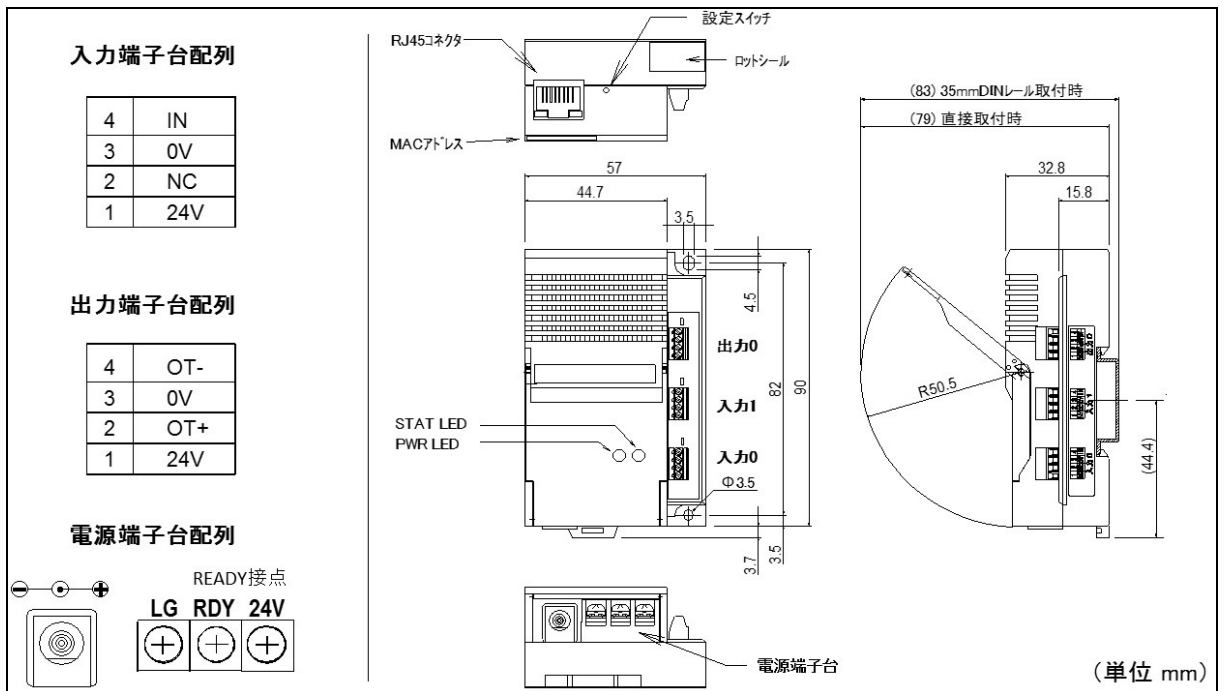
図 3-2-2 UNC-RP31CTA 外形寸法図
