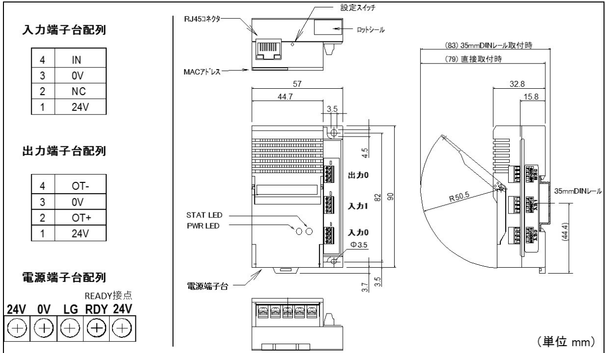
図 3-2-1 UNC-RP31CT 外形寸法図
