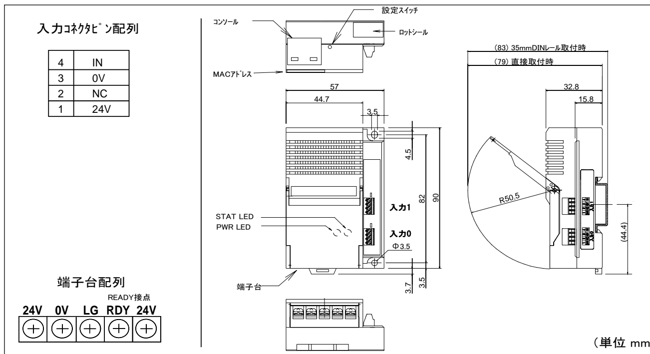
図 2-2-1 UNC-WRP06 外形寸法図
