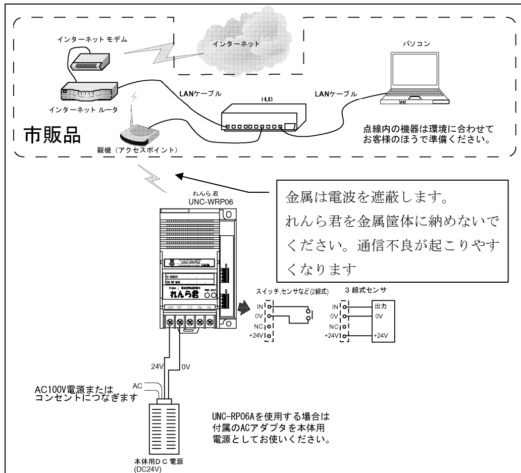
図 2-2-3 れんら君の接続図
