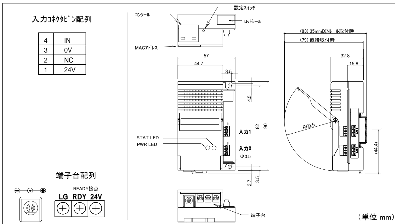
図 2-2-2 UNC-WRP06A 外形寸法図
