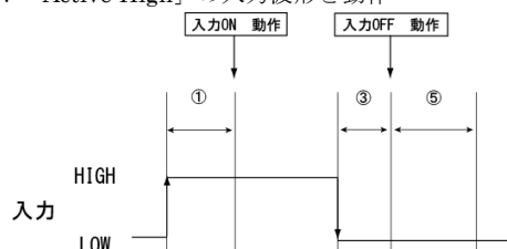
図 2：「Active High」の入力波形と動作
