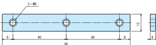
トリプルナット 型式 OPS1-8
