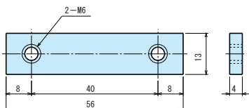
ダブルナット 型式 OPS1-7
