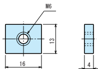
M6ナット 型式 OPS1-5
