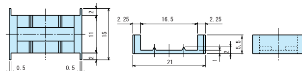
ナット固定ゴム 型式 OPS1-9
