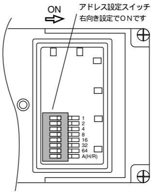
アドレス設定スイッチ
